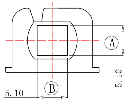
A-A SECTION
