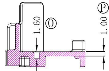
SEC. A-A
