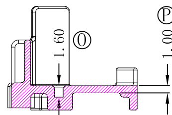
SEC. A-A
